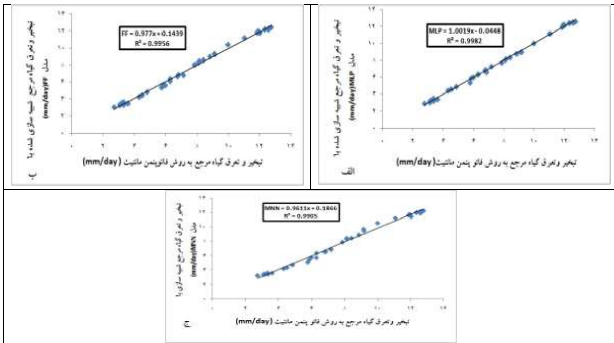
شکل ۴: مقایسه تبخیر و تعرق گیاه مرجع محاسبه شده با روش فائوپنمن مانتیث با سه شبکه MLP (الف)، FF (ب) و MNN (ج) در سناریو چهارم.
